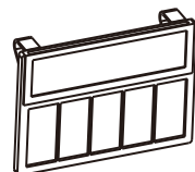
产品名称：数字价格翻牌 Product Name: Price Cassette 材质：ABS Material: ABS 规格：123x85mm Size: 123x85mm 颜色: 黑色/红色/蓝色 Color: Black/red/blue 型号：105060001 Code: 105060001
