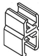
产品名称: 框对框连接件 Product Name: Frame Connector 材质: PC Material: PC 颜色: 透明 Color: Clear 型号: 302008 Code: 302008
