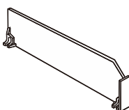
名称: T形分隔板 Product Name: Shelf Divider with T front 材质: PC Material: PC 规格: 60mmx(185/485)mm 120mmx(185/485)mm Size: 60mmx(185/485)mm 120mmx(185/485)mm 颜色: 透明 Color: Clear 型号: 201008 Code: 201008
