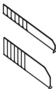
名称: 可折断分隔板 Product Name: Breakable Divider 材质: PET Material: PET 规格: 60mmx(185/485)mm 120mmx(185/485)mm Size: 60mmx(185/485)mm 120mmx(185/485)mm 颜色: 透明 Color: Clear 型号: 201024 Code: 201024
