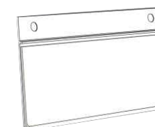
产品名称: 标签槽 BH Product Name:Data Strip BH 材质: PVC Material:PVC 规格: 39/60/80/90mm Size:39/60/80/90mm 颜色:透明 Color:Clear 型号: 101005 Code:101005
