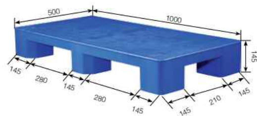
名称: 64#平面六角卡板 Product Name: 64# Flat Pallet 材质: PP Material: PP 规格: 1000x500x145 Size: 1000x500x145 颜色: 黑色/蓝色 Color: Black/blue
